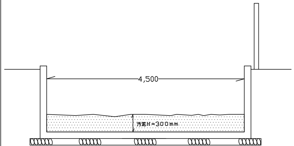
標準断面図 1/50 A-A'
