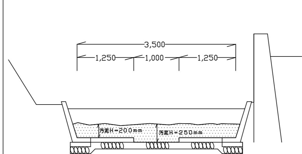
標準断面図 1/50 B-B'
