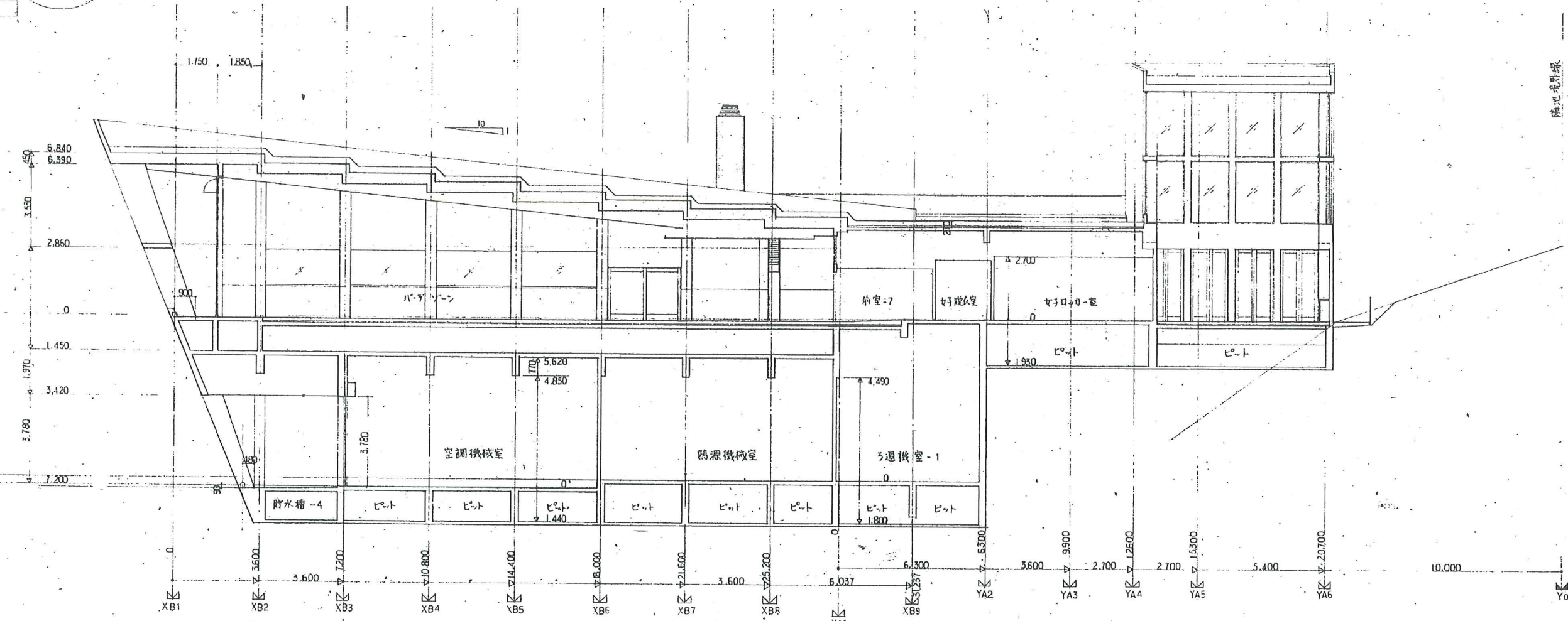
B線 e-e' 断面図 1:100
