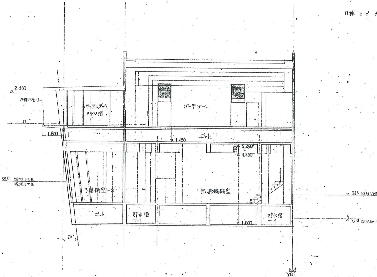
B線 f-f' 断面図 1:100
