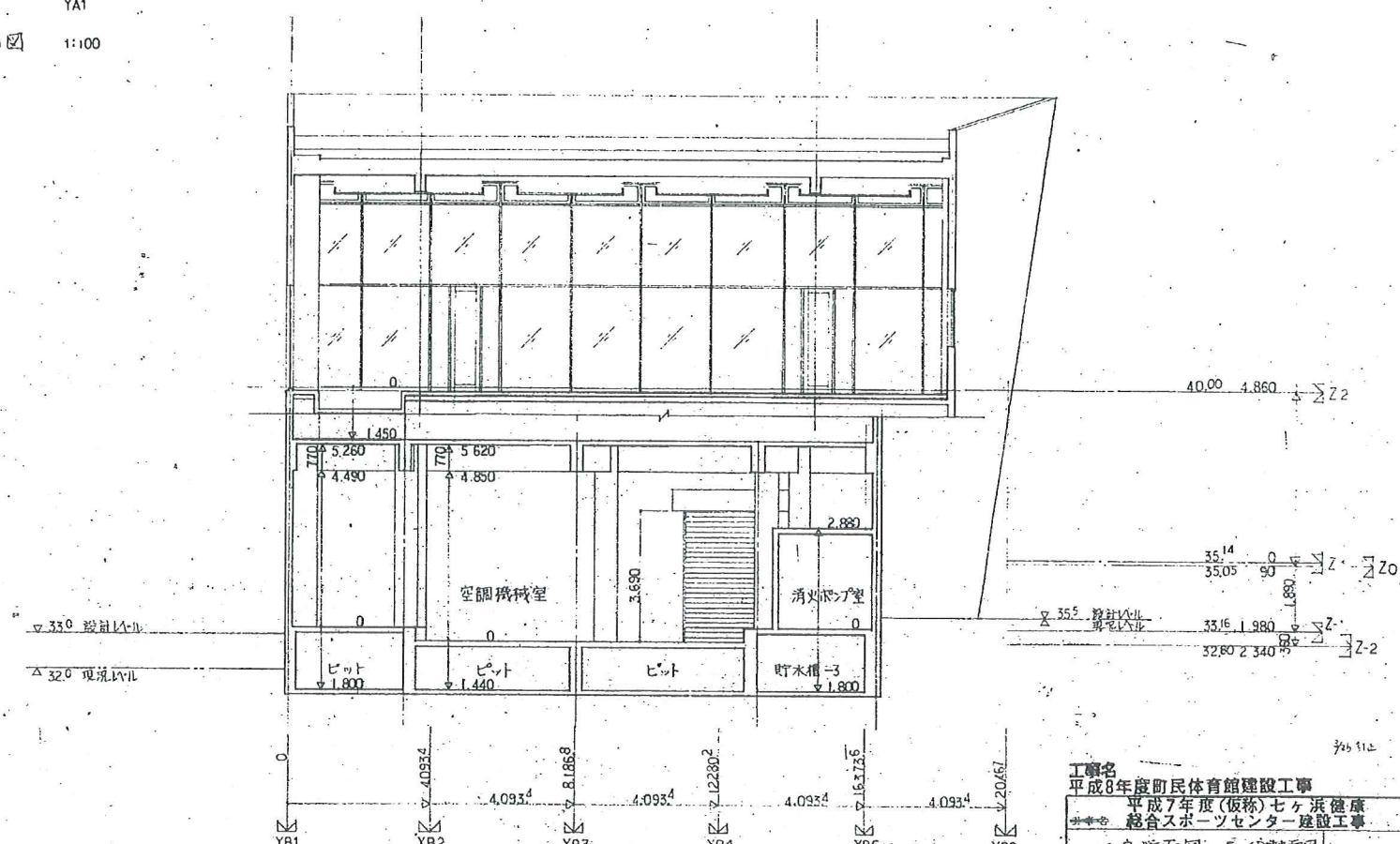
B線 g-g' 断面図 1:100
