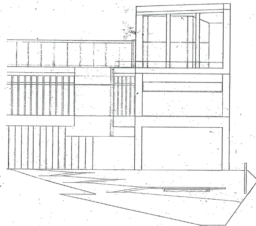
広場-1 南側立面図 S-1:100
